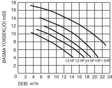
PERFORMANS EĞRİLERİ
