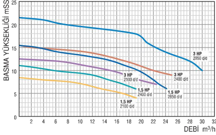
DEĞİŞKEN HIZLI MOTOR PERFORMANS EĞRİLERİ
