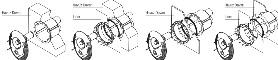
Beton Yüzme Havuzu
