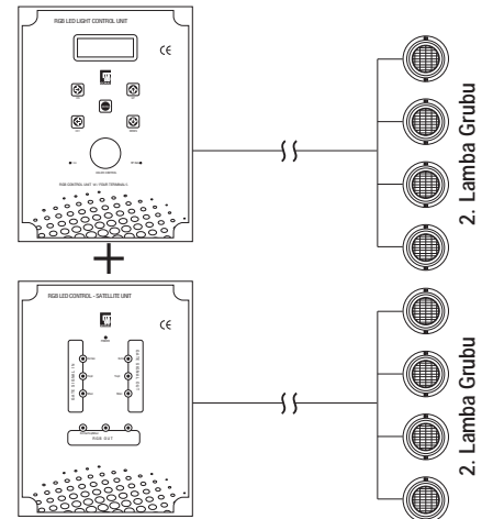
Merkezi Kumanda Panosu 05073221/05073222
