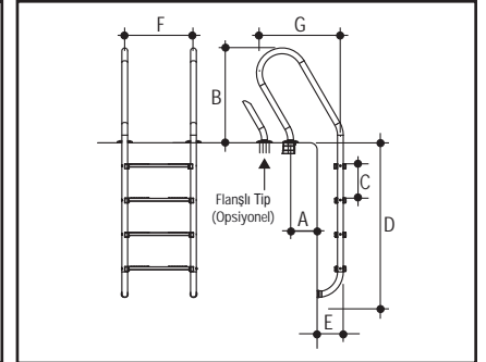
KOMBİNE
