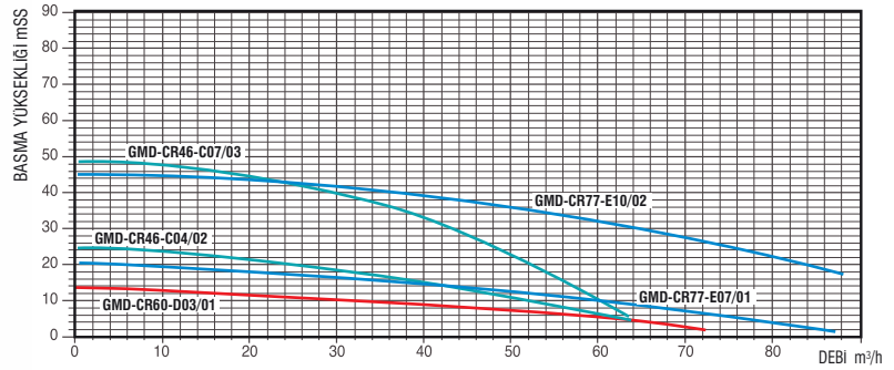
PERFORMANS EĞRİLERİ
