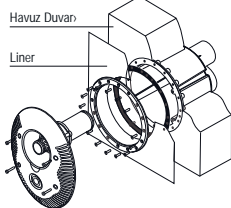
Liner Yüzme Havuzu
