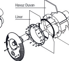
Liner Panel Yüzme Havuzu
