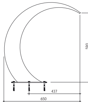
Yandan görünüş
