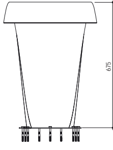
Önden görünüş
